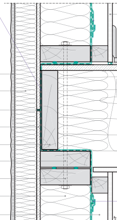
Coupe verticale
